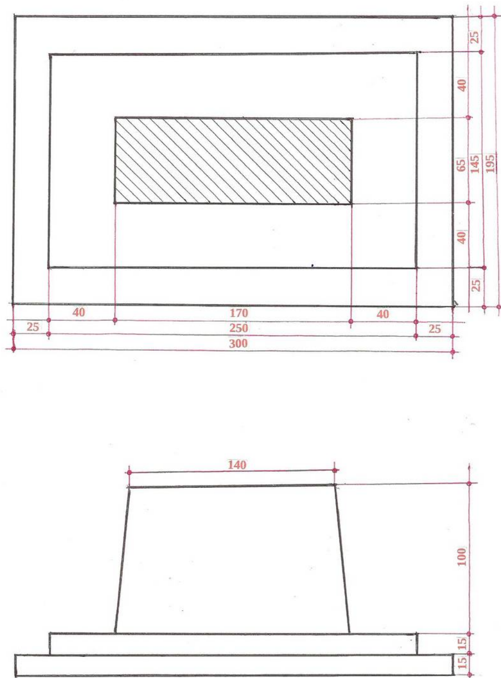
PODEST POMNIKA /wymiary podane w cm/
